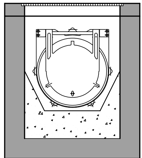
Schnitt B-B
